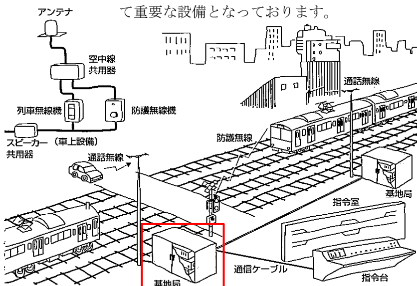
図 列車無線設備システム概要（イメージ図）
